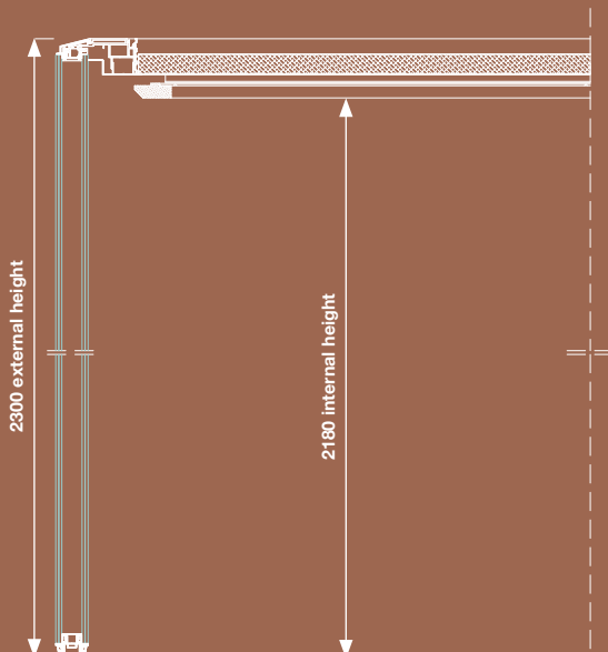
Sezione verticale Vertical section Section vertical Seccion vertical
